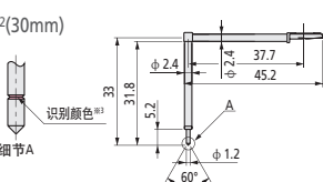
深槽用 ※2(30mm)
