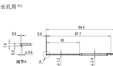
细长孔用 ※2
