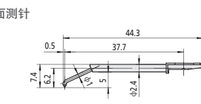
孔底面测针
