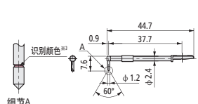
刀刃用
