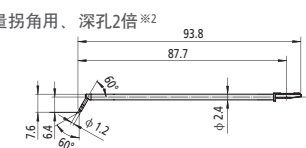
孔底面测针
