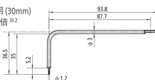
深槽用 (30mm)
