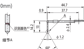
深槽用 ※2(20mm)
